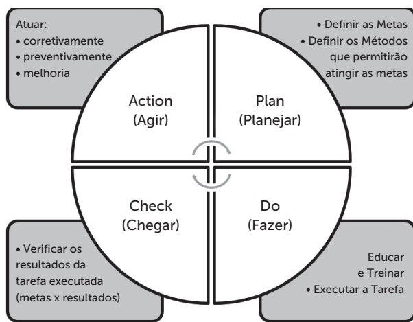
Figura 3.7 | Ciclo PDCA
